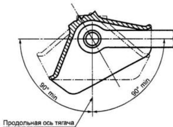
Рисунок 5 - Поворот сцепленной проушины сцепной тяги по горизонтали
