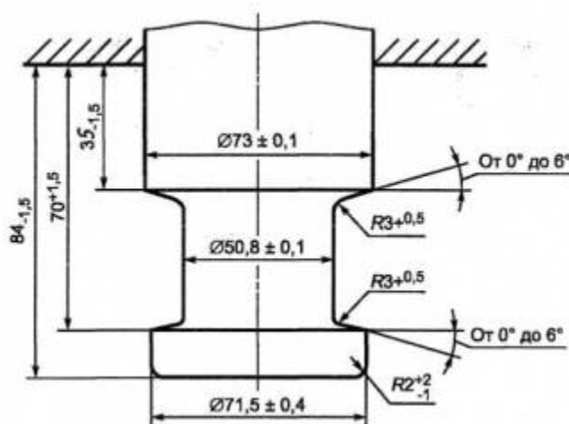
Рисунок 18 - Размеры шкворней седельно-сцепных устройств класса Н50
