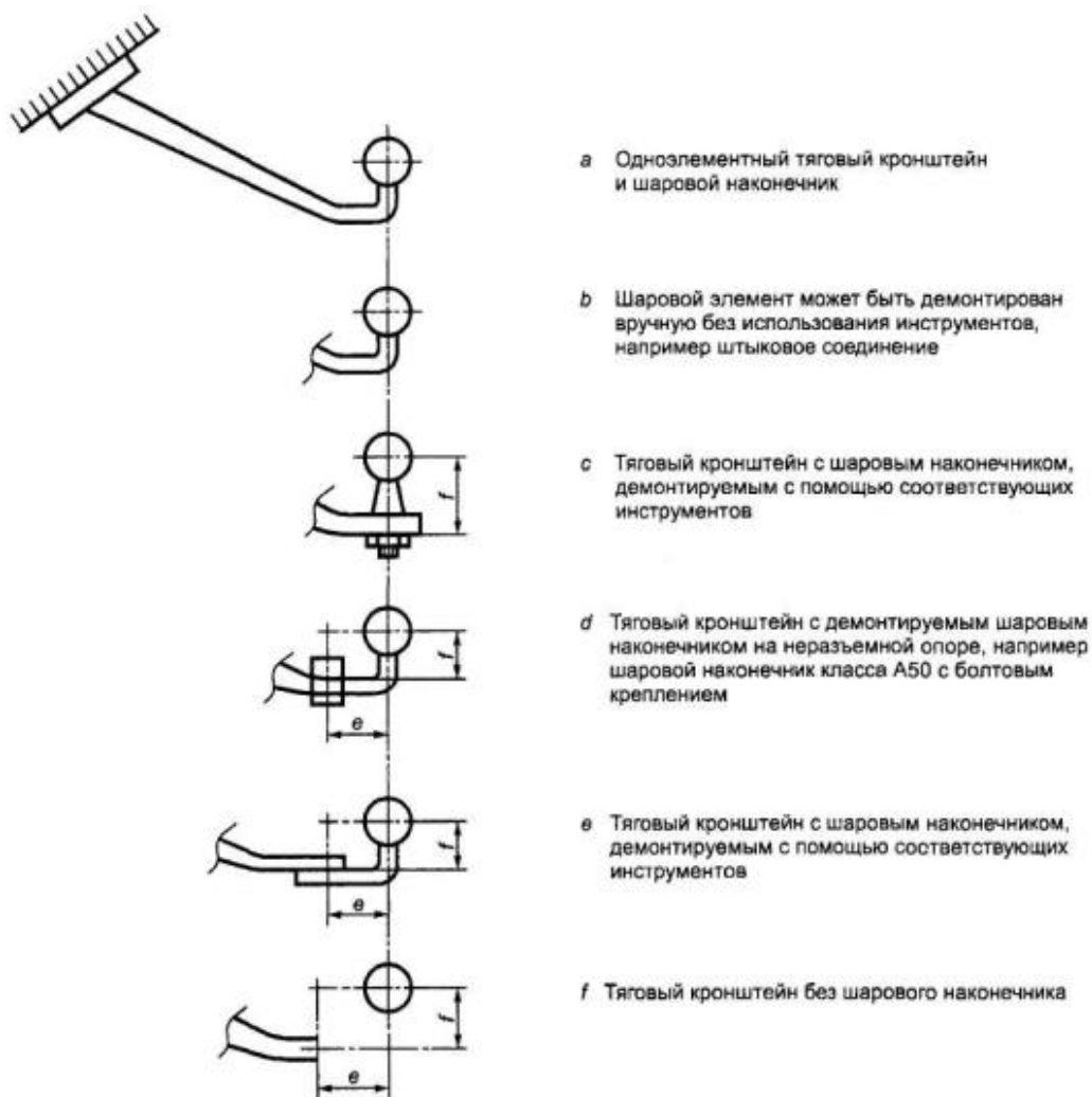
Рисунок 20 - Схема тяговых кронштейнов шарового типа
