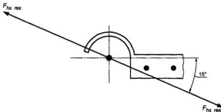
Рисунок 23 - Динамическое испытание
