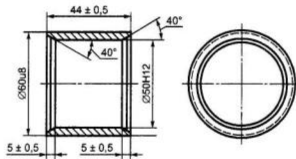
Рисунок 10 - Втулка без прорези для проушин сцепных тяг класса D50-C
