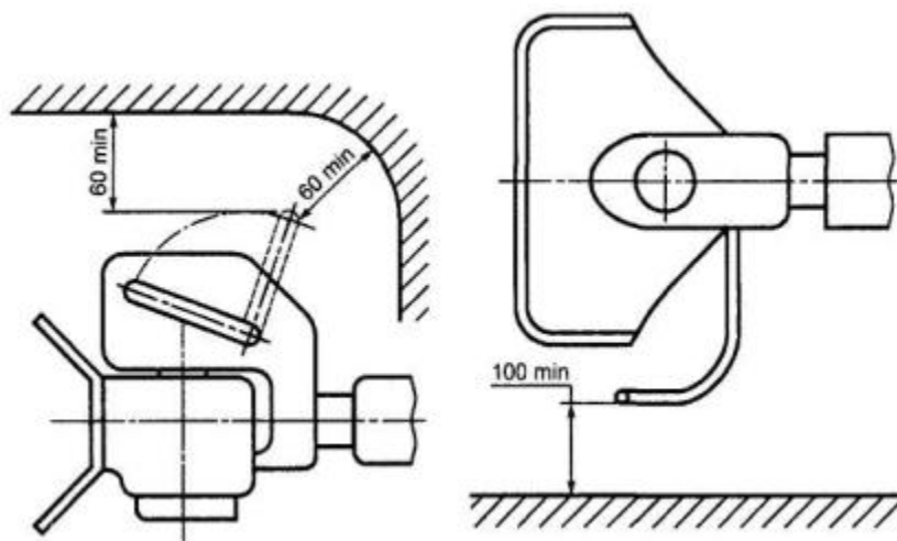
Рисунок 26 - Свободное пространство рукоятки
