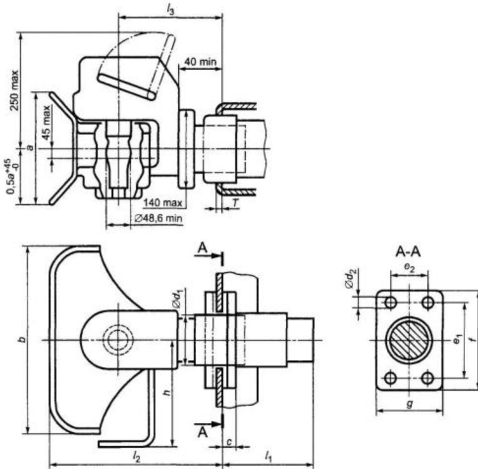
Рисунок 8 - Размеры стандартных соединительных фланцев сцепных тяг
