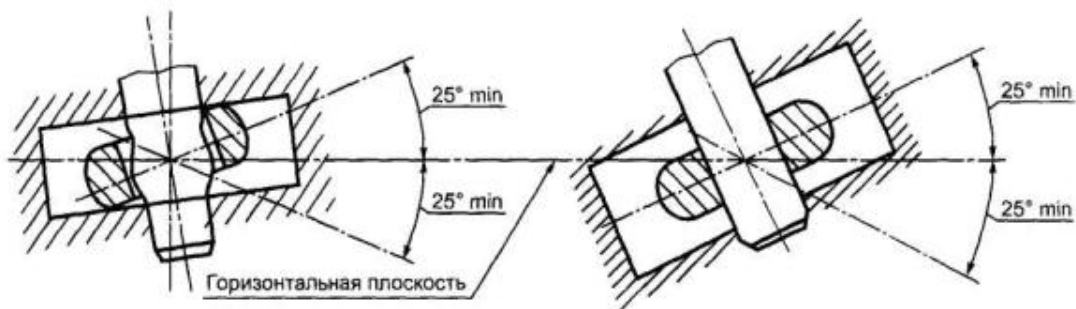
Рисунок 7 - Поворот сцепленной проушины сцепной тяги вокруг оси
