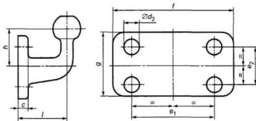
Рисунок 4 - Размеры стандартных фланцевых шаровых наконечников классов А50-2 - А50-5
