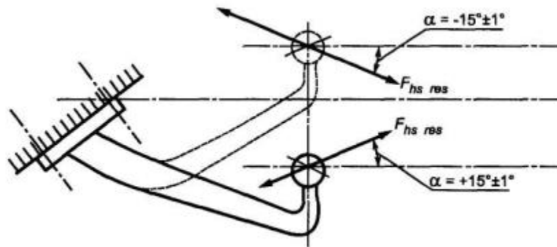
Рисунок 21 - Углы приложения испытательной силы
