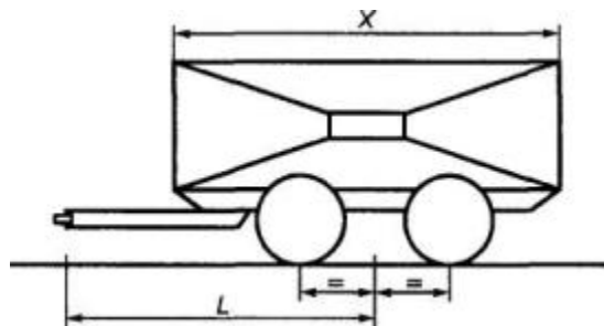
Рисунок 1 - Габаритные размеры прицепа с центральной расположенной осью
